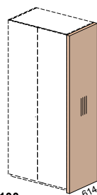
52H100 50x614x2261 (1 шт.)
