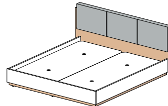
52K021 без матраца 2038x2076x896
